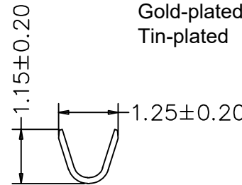
剖视图: B-B
