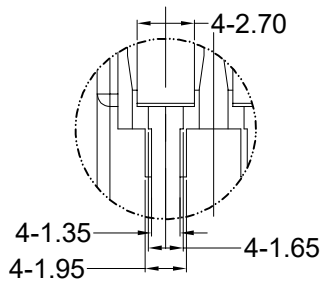
局部视图 C 比例 3:1
