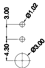
2P P.C.B LAYOUT
