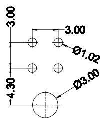
4P~6P P.C.B LAYOUT
